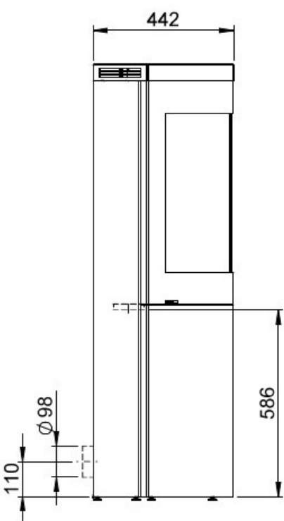
Maße: externe Zuluft
