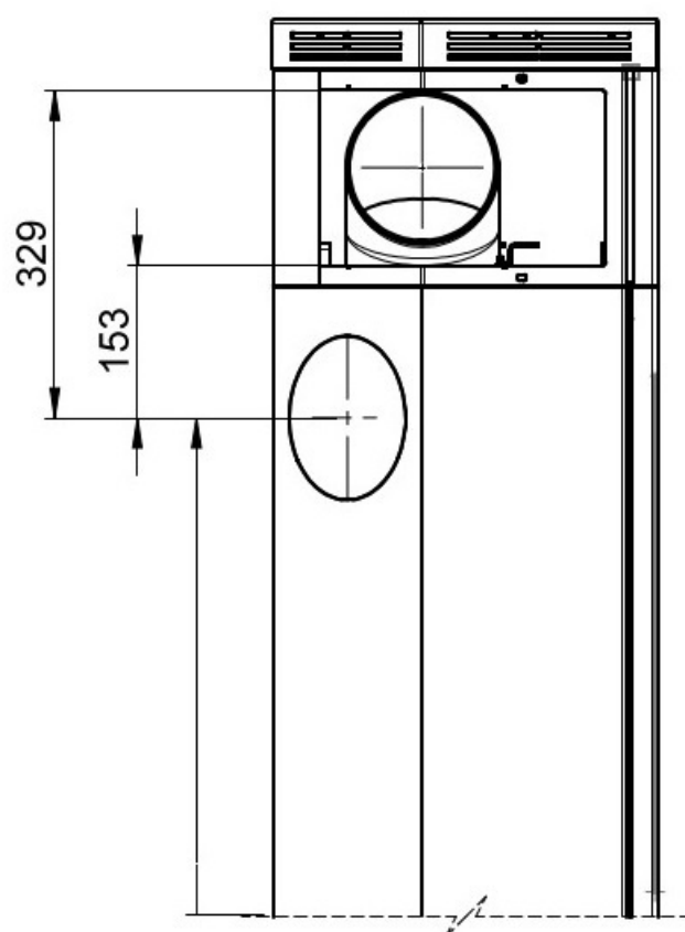
Maße: seitlicher Rauchausgang
